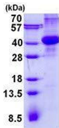
15% SDS-PAGE (3µg)
