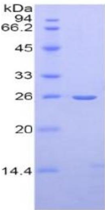
15% SDS-PAGE
